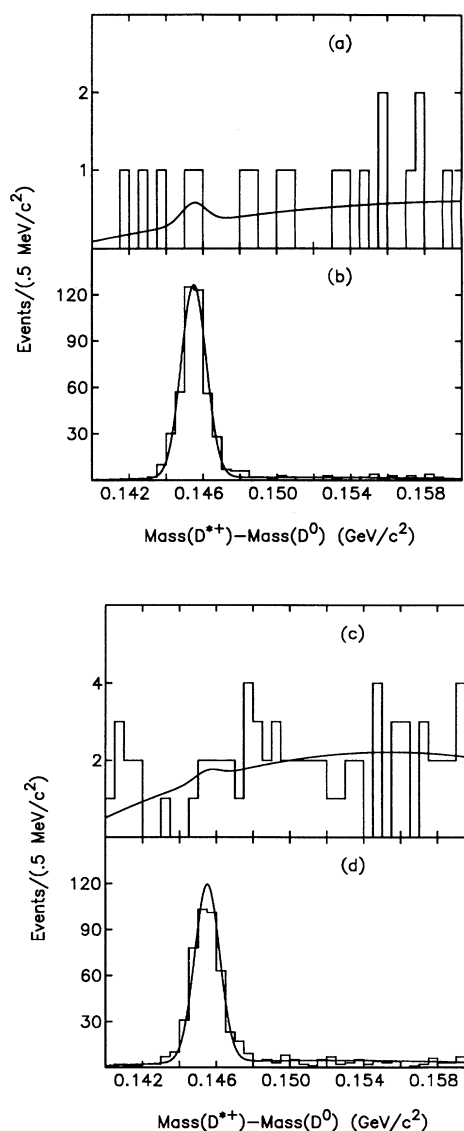
FIG. 4. (a) D^{*+}-D^0 mass-difference plots for (a) D^0 \rightarrow K^+\pi^- , (b) D^0 \rightarrow K^-\pi^+ , (c) D^0 \rightarrow K^+\pi^-\pi^+\pi^- , and (d) D^0 \rightarrow K^-\pi^+\pi^-\pi^+ .
